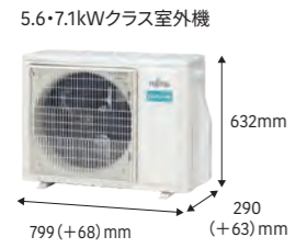
対応風向ガイド(別売) [OP-J02B] ※室外機の外寸算出の際には( )内の寸法をプラスしてください。
