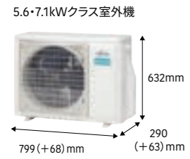
対応風向ガイド(別売) [OP-J02B] ※室外機の外寸算出の際は( )内の寸法をプラスしてください。
